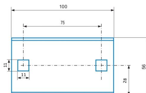
príruba KBB
